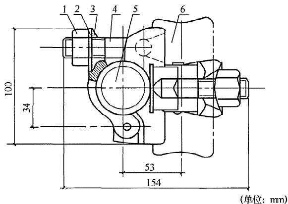
图 6 直角扣件
