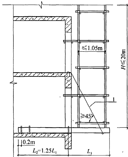
图 6.10.2 型钢悬挑脚手架构造
