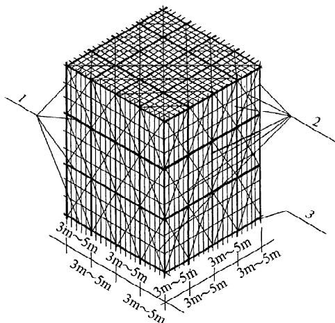
图 6.9.3-2 加强型水平、竖向剪刀撑构造布置图
