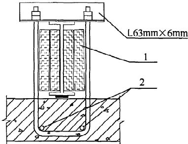
图 6.10.5-1 悬挑钢梁 U 形螺栓固定构造
