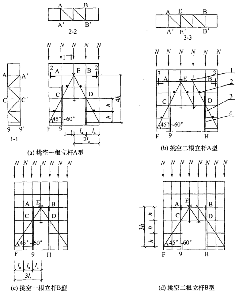
图 6.5.1 门洞处上升斜杆、平行弦杆桁架
