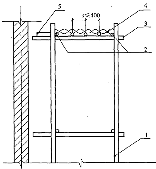
图 6.2.1-2 铺竹笆脚手板时
