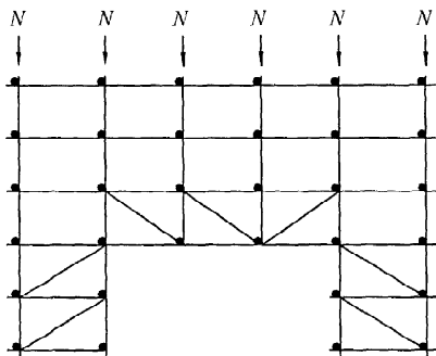
图 9 英、法等国过门洞的结构形式
