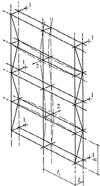
图 7 双排脚手架的整体失稳 1—连墙件；2—失稳方向
