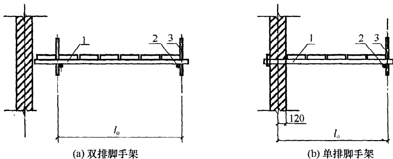
图 5.2.4 横向水平杆计算跨度
