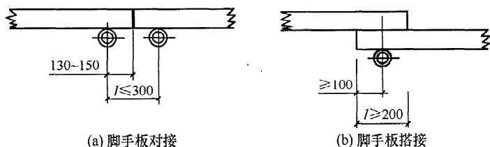
图 6.2.4 - 脚手板对接、搭接构造
