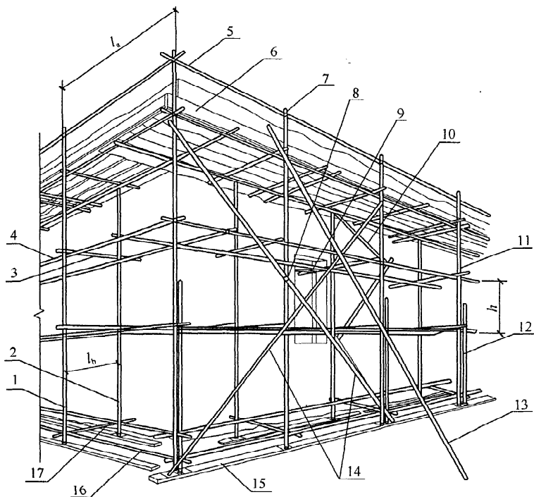
图 1 双排扣件式钢管脚手架各杆件位置
