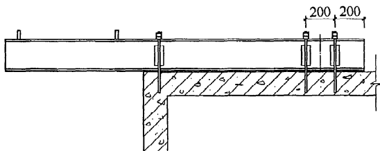
图 6.10.5-3 悬挑钢梁楼面构造
