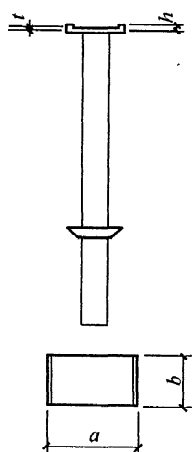
图 3 可调托撑构造图
