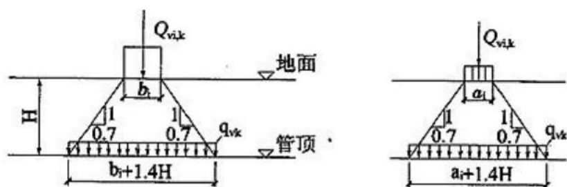
(a) 顺轮胎着地宽度的分布
