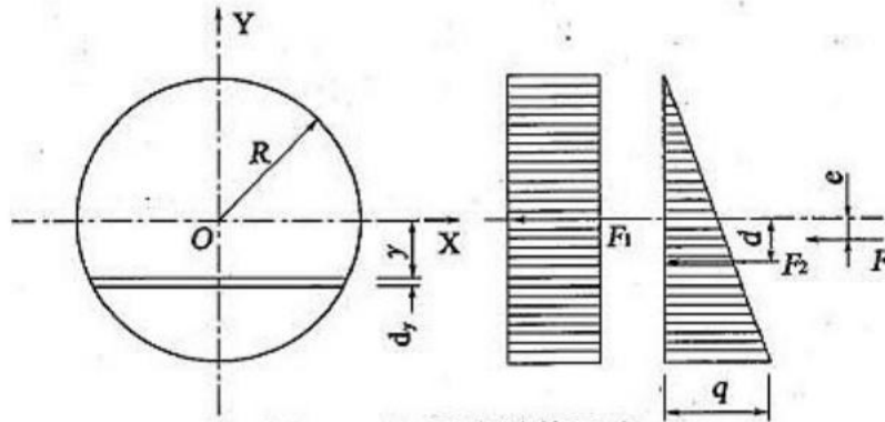
图4 正面阻力计算图式
