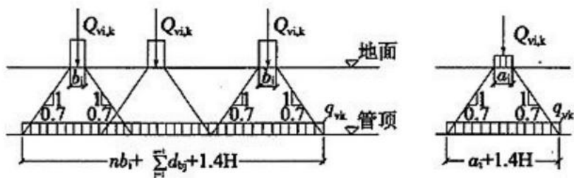
(a) 顺轮胎着地宽度的分布
