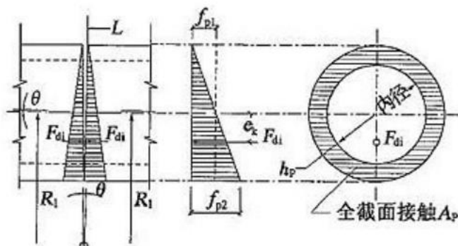
图5. 5. 4-1 不张口接头的受力模式
